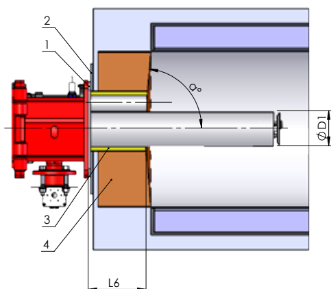
Quemador Low NOx LN30
