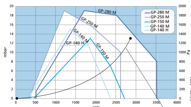
Gráfico de pérdida de presión de la caldera en función de la capacidad del quemador.
